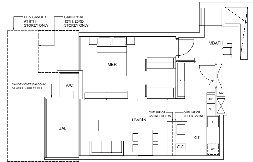
TYPE A2 55 sqm / 592 sqft
