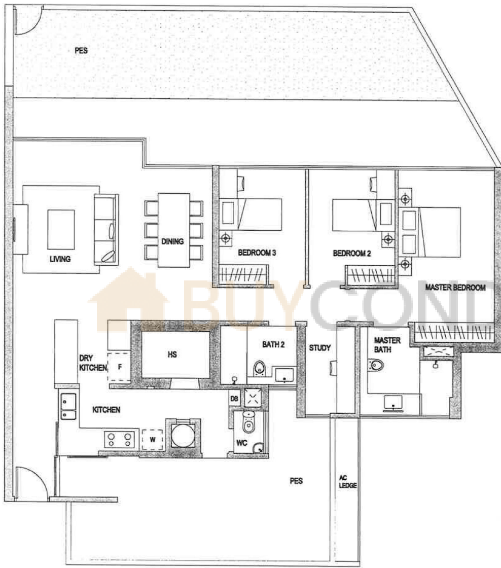
TYPE F1(P3) : 3-BEDROOM + STUDY — sq m/ —sq ft #01-34
