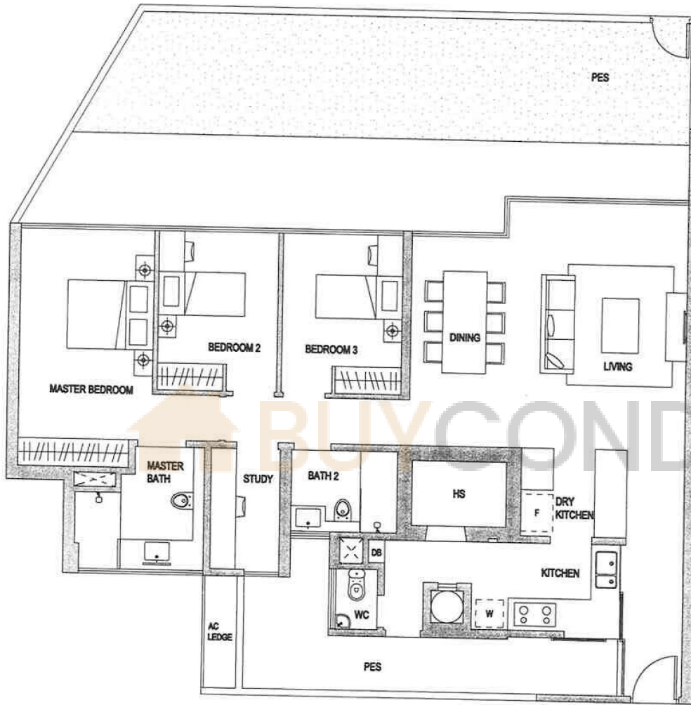
TYPE F1(P2) : 3-BEDROOM + STUDY — sq m/ —sq ft #01-29, #01-33
