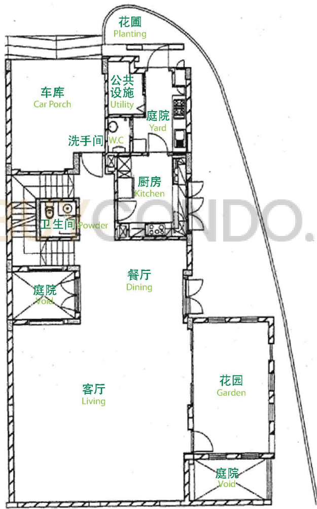
1 st Storey Floor Plan 第一层平面图
