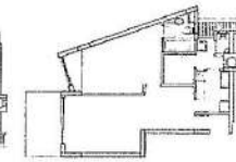
D15 - 71 sqm Living & Dining - 25.75 sqm Master Bedroom - 16.30 sqm
