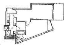
D13 - 68 sqm Living & Dining - 23.70 sqm Master Bedroom - 16.30 sqm
