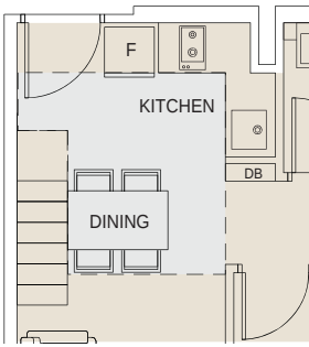
LOFT UNIT
