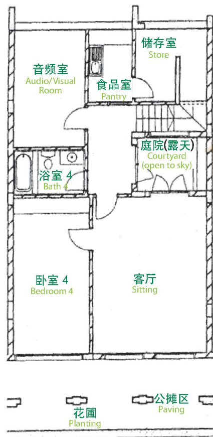
Basement Floor Plan 地下室平面图
