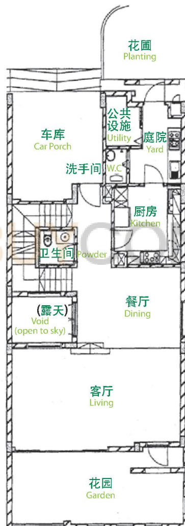
1 st Storey Floor Plan 第一层平面图
