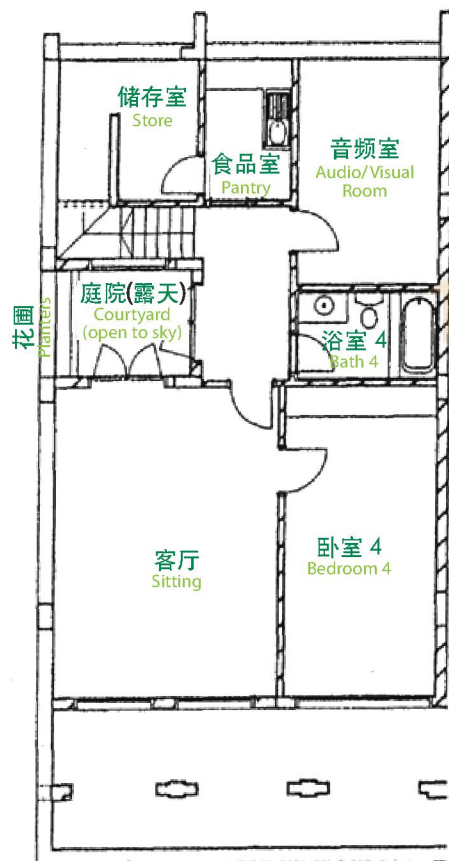
Basement Floor Plan 地下室平面图
