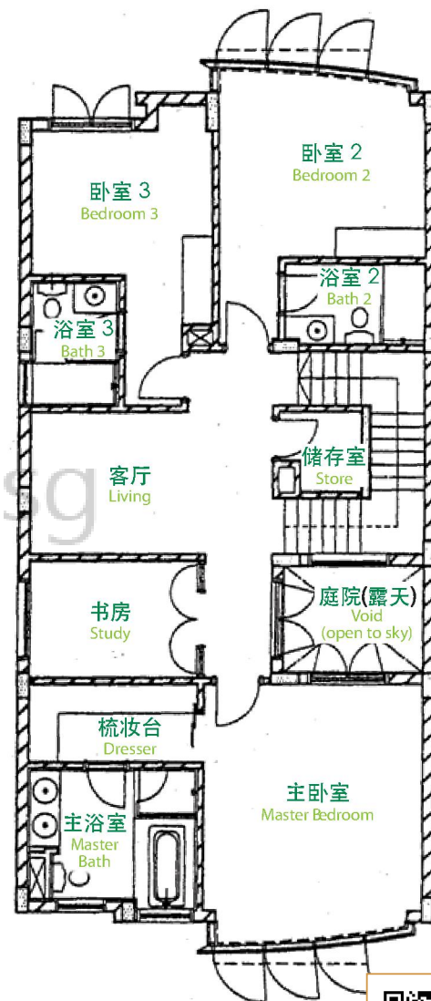
2 nd Storey Floor Plan 第二层平面图
