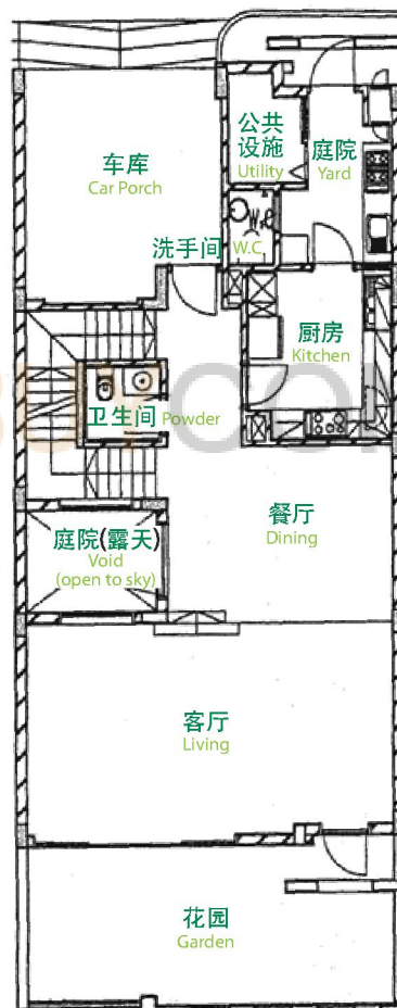
1 st Storey Floor Plan 第一层平面图
