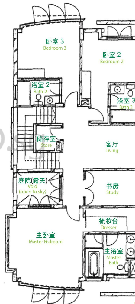
2 nd Storey Floor Plan 第二层平面图
