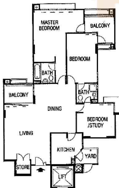
TYPE F3
