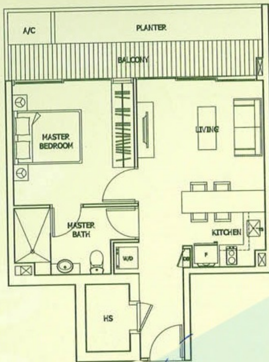
TYPE A4 #02-09 - #04-09
