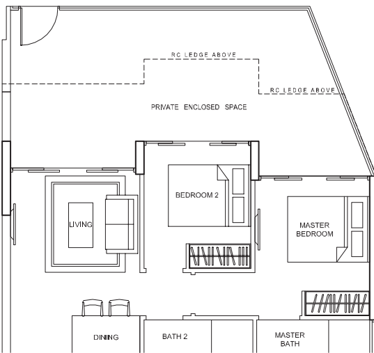
TYPE B3aP2 Area : 95 sq.m Unit : #01-39 (mirror image)
