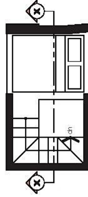
LOFT PLAN
