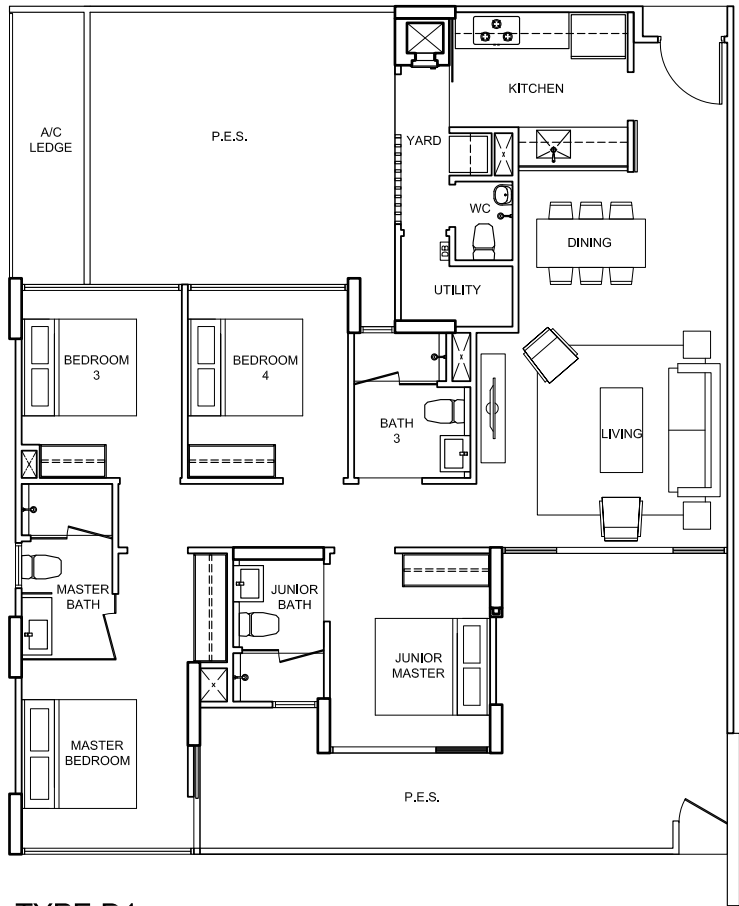
TYPE D1-pes 164 sqm/ 1,768 sq ft 88, Elias Road # 01 - 27
