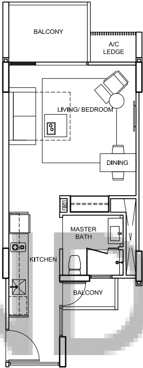
TYPE A5 44 sqm/ 475 sq ft 98, Elias Road # 05 - 60 # 04 - 60 # 03 - 60 # 02 - 60
