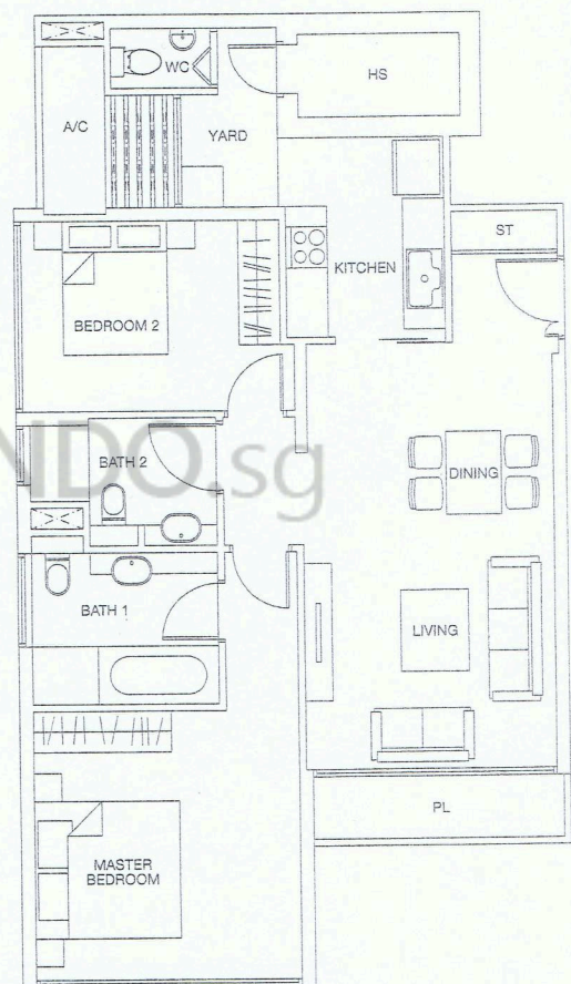
TYPE A2-a
