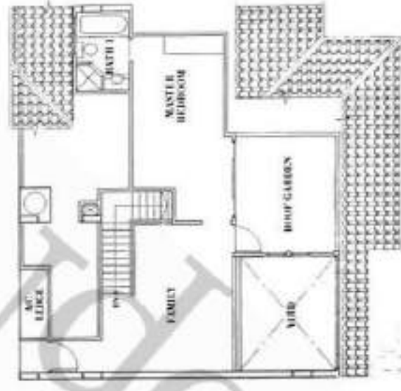
Type E4 (b)
