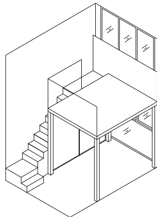
AXONOMETRIC
